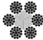
6x25F
